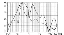
250A (FMAC-0956-H312I)
