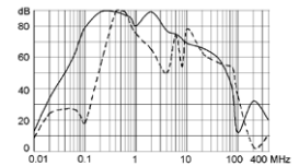
64A (FMAC-0953-6412I)
